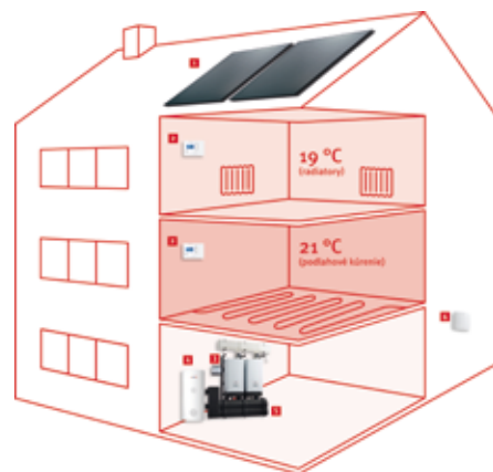
Schéma zapojenia kaskády v dome.
